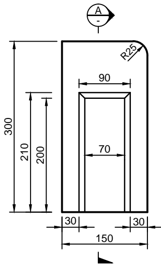
END ELEVATION
